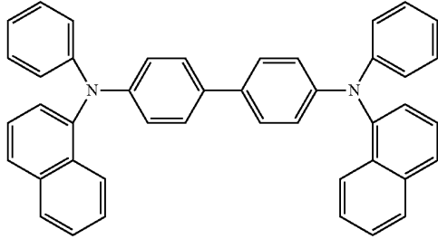
a-NPD
