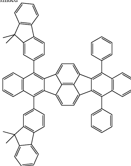
B-1
