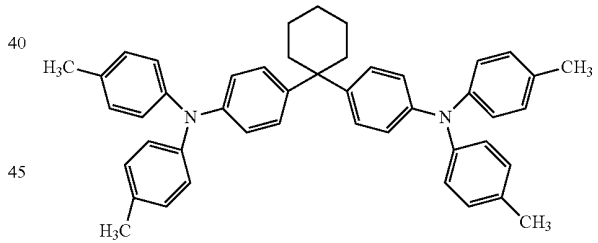
TPAC
