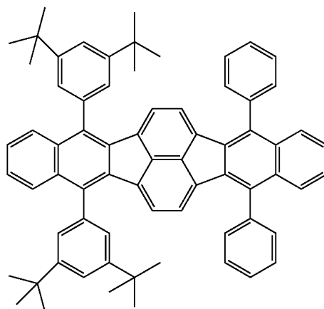
B-20
